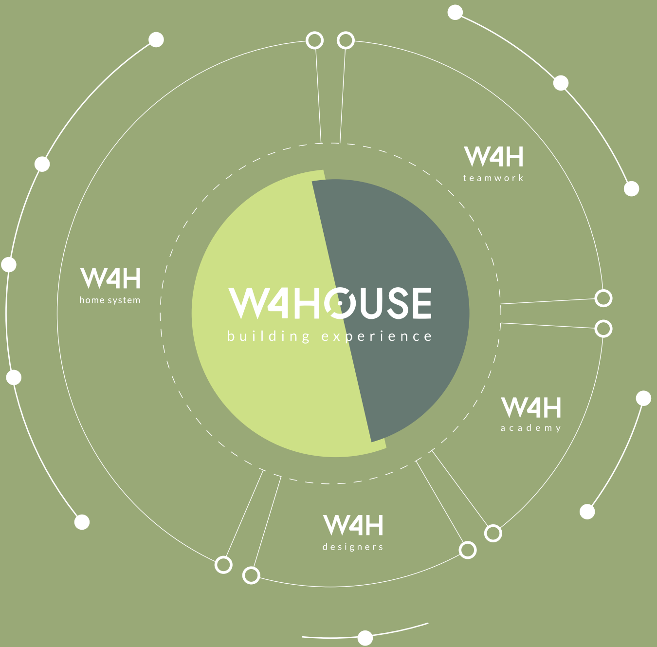
Mapa di inquadramento dell'universo W4H
