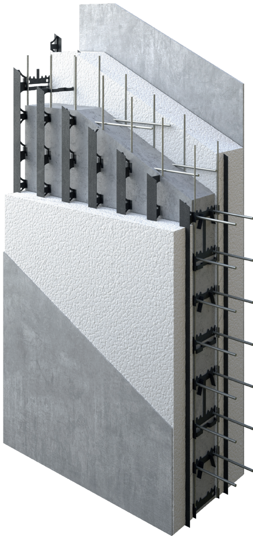
Sistema parete, tipologia Setto.
